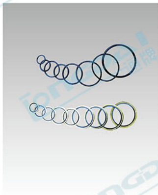
JB982-77组合密封垫圈、仿进口型 JB982-77 Semimetallic Gasket、 Fake Imported Type 公称口径nominal Dia: Φ6-Φ60mm 压力等级pressure Grade:40MPa 工作温度working temperature: -25℃+80℃
